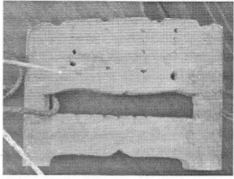
Fyra resonanssträngar verkar ha legat mellan nyckelraderna, resten är placerade under nycklarna. Översadeln har motsvarande hål och uttag.
